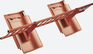
Aluminijasta snegolovna rešetka
